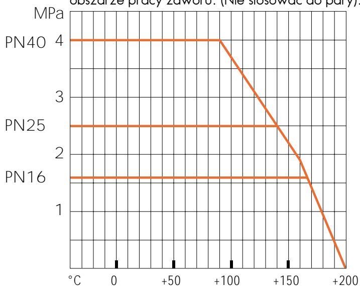
Wykres zależności (ciśnienie/temperatura) w obszarze pracy zaworu. (Nie stosować do pary).
